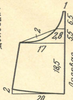
Карман, (Мод. №2) 2 дет.
